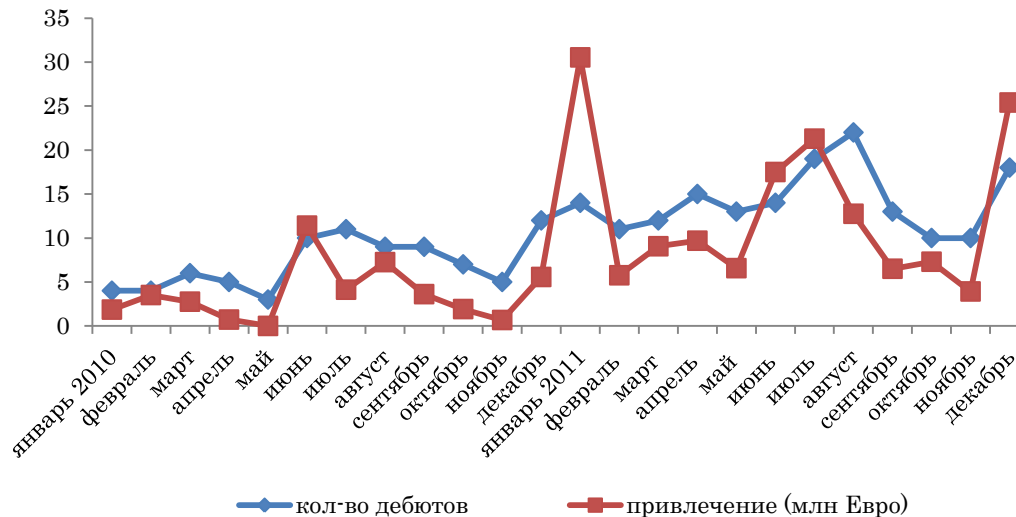
Рис. 2. Количество дебютов и объёмы привлечения на рынке NewConnect
